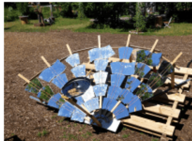
Selbstbau-Parabolspiegel gebrauchte Spiegel 1.5m 2 (15 €), Glasschneider (10 €), gebrauchter Lattenrost 140 cm (20 €), mit Kleinkram insgesamt ca. 50 €
